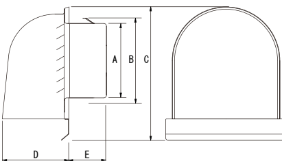
■寸法図
