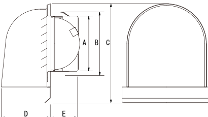
■寸法図
