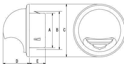
■寸法図
