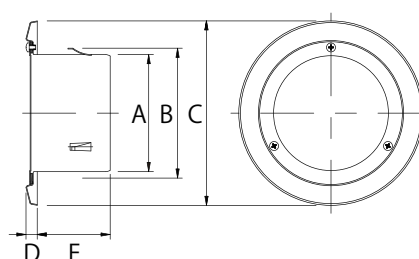
■寸法図
